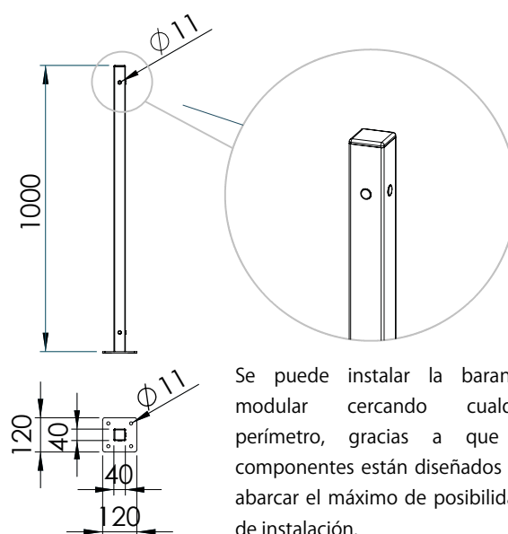
POSTE ATORNILLAR
